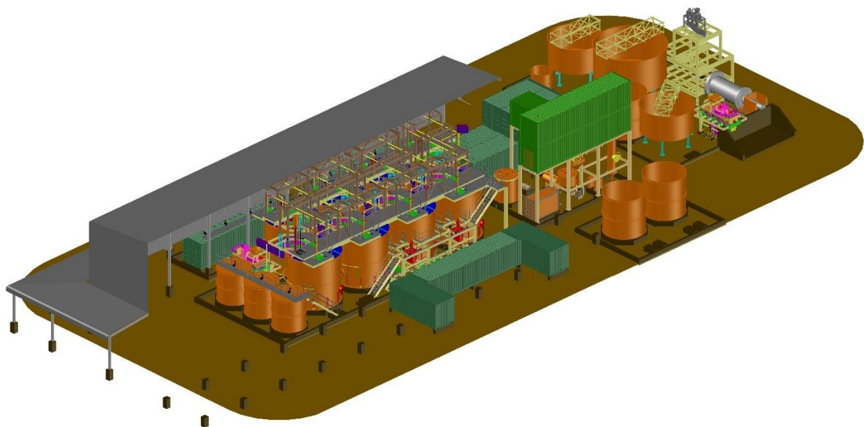
Plan 3D de la future usine de cyanuration de Dieu Merci.
